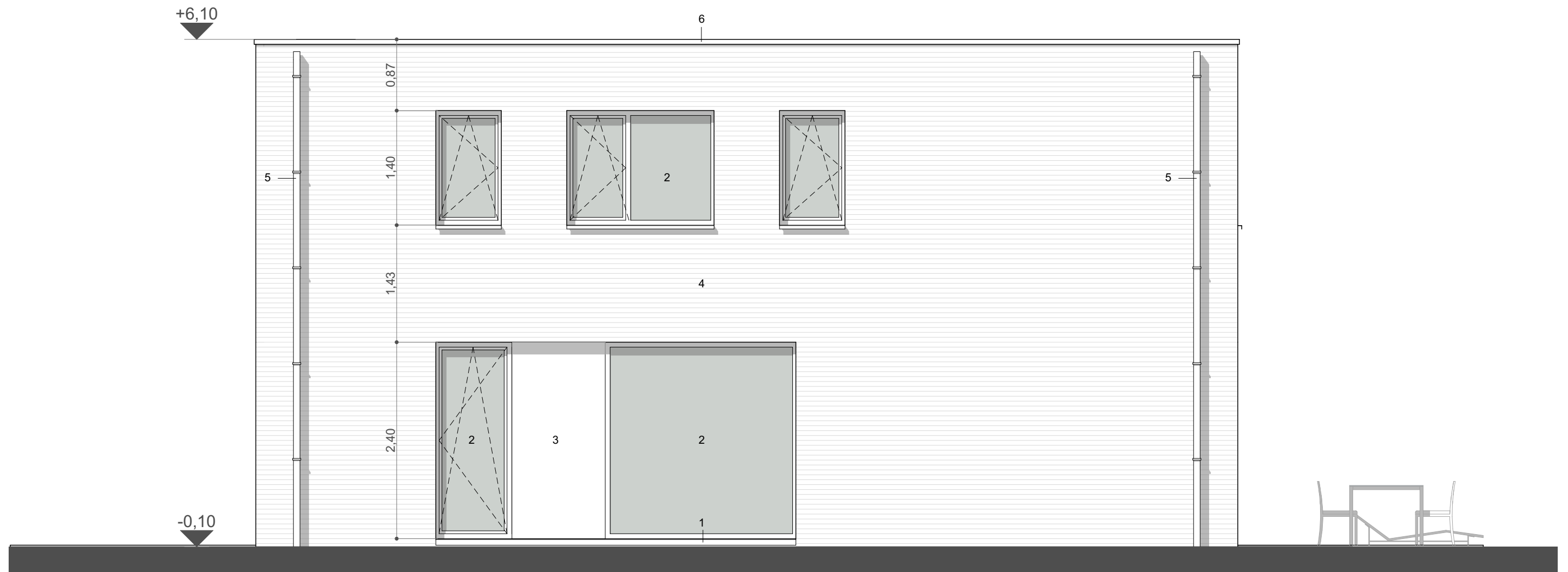
ZIJGEVEL RECHTS 1/50
